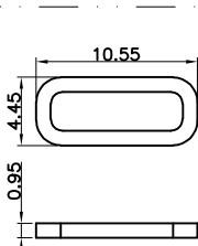
防水圈图示
